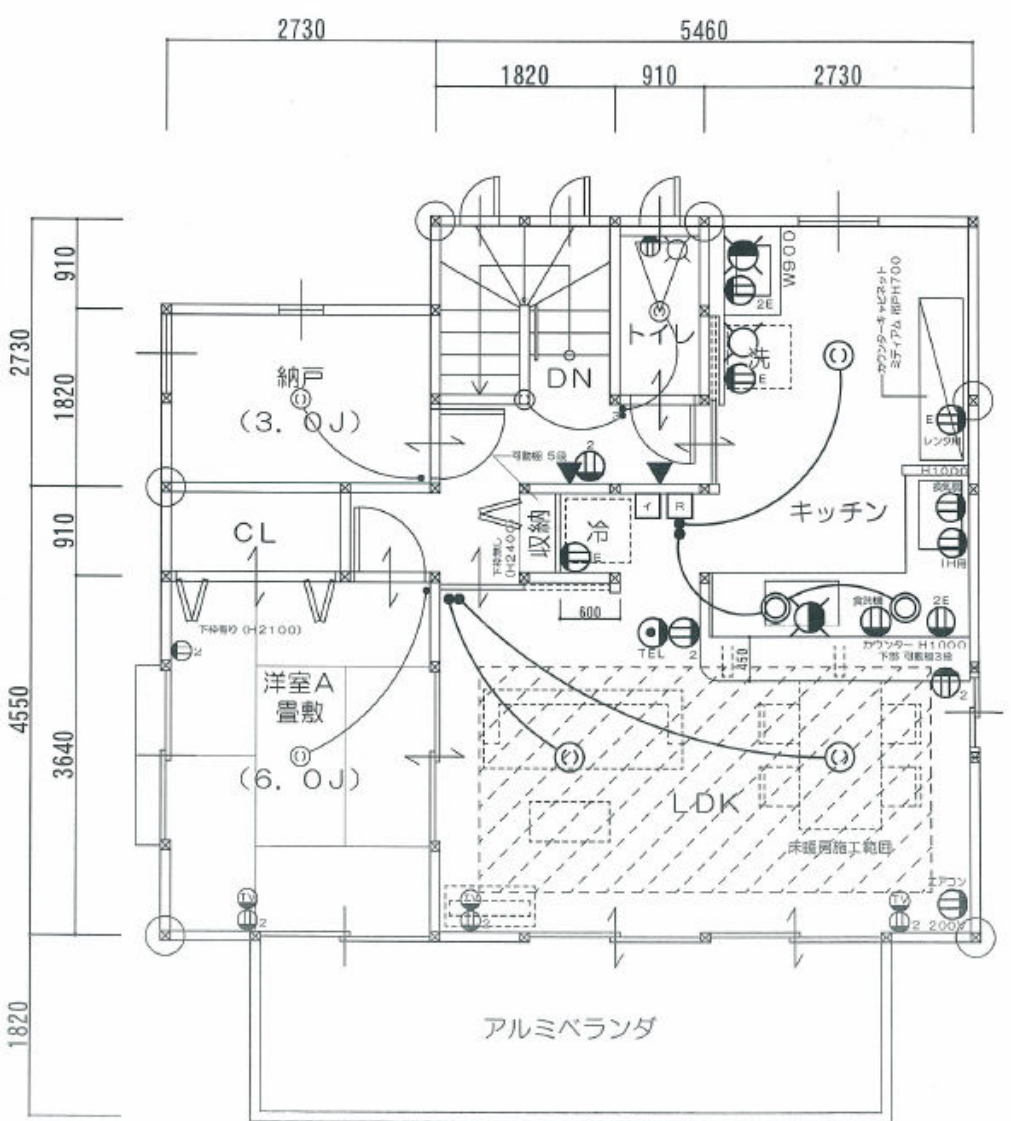
2F プラン図
