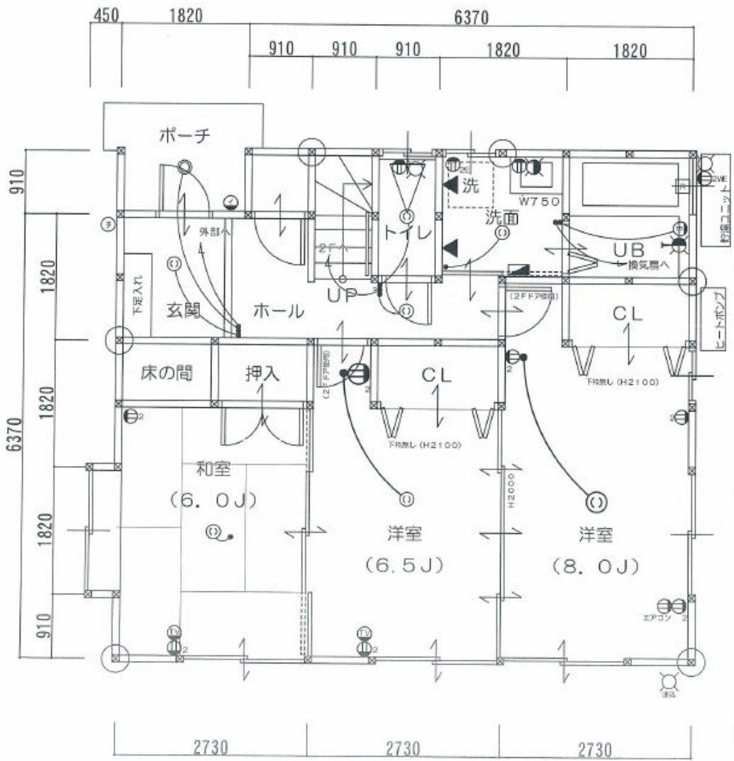
1F プラン図
